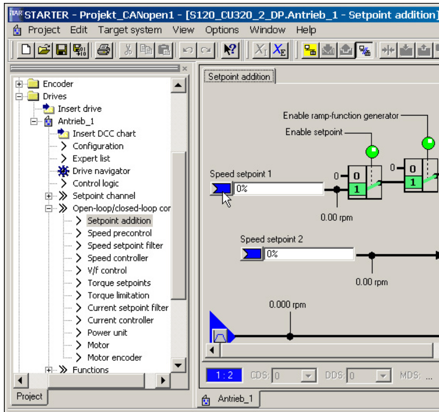
Изображение 3-7 Суммирование заданных значений
