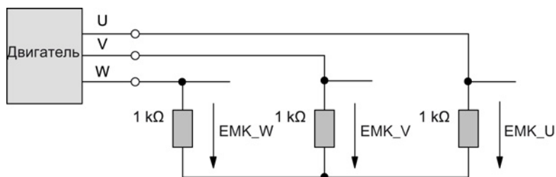
Изображение 3-56 Расположение для контрольного измерения
