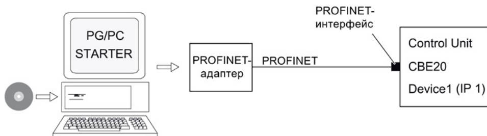
Изображение 3-19 Соединение программатора с целевым устройством через PROFINET (пример)
