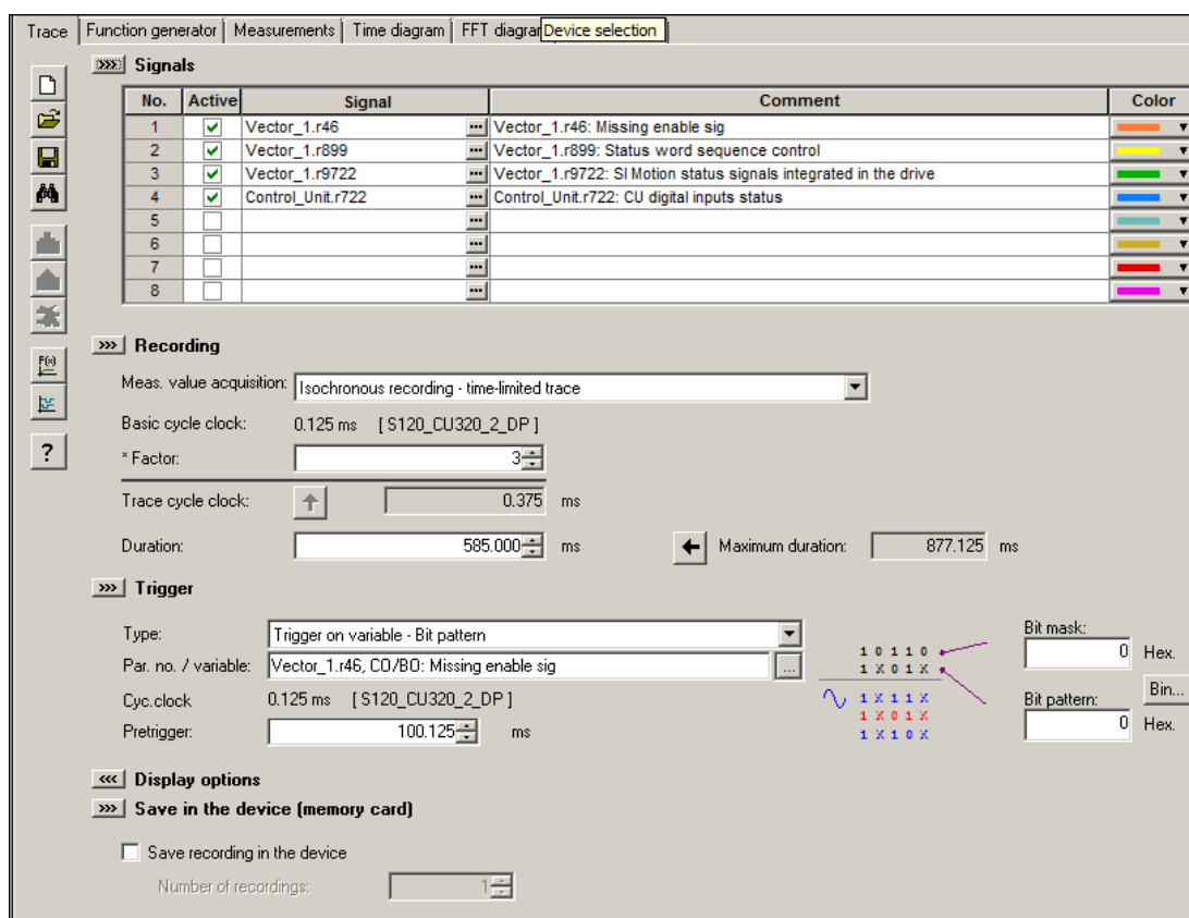
Изображение 4-6 Многократная трассировка в STARTER
