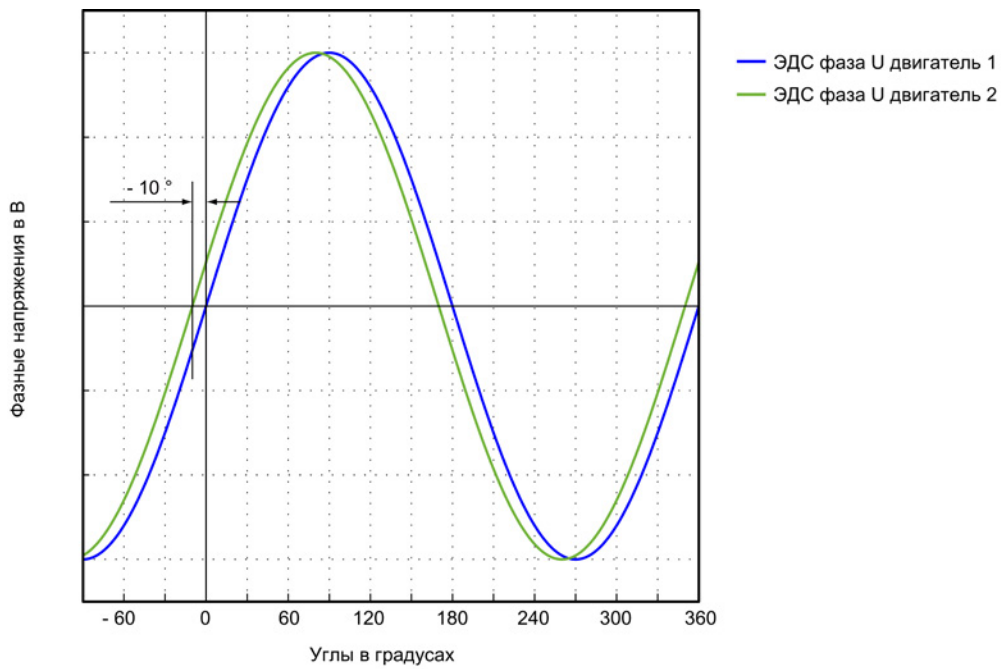
Изображение 3-58 Фаза U двигателя 1 может отставать от ЭДС фаза U двигателя 2 не более чем на 10^\circ
