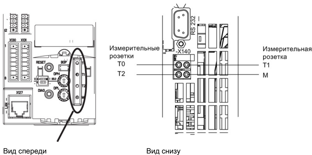
Изображение 4-11 CU310-2 DP/PN измерительные розетки, CU320-2 DP/PN измерительные розетки
