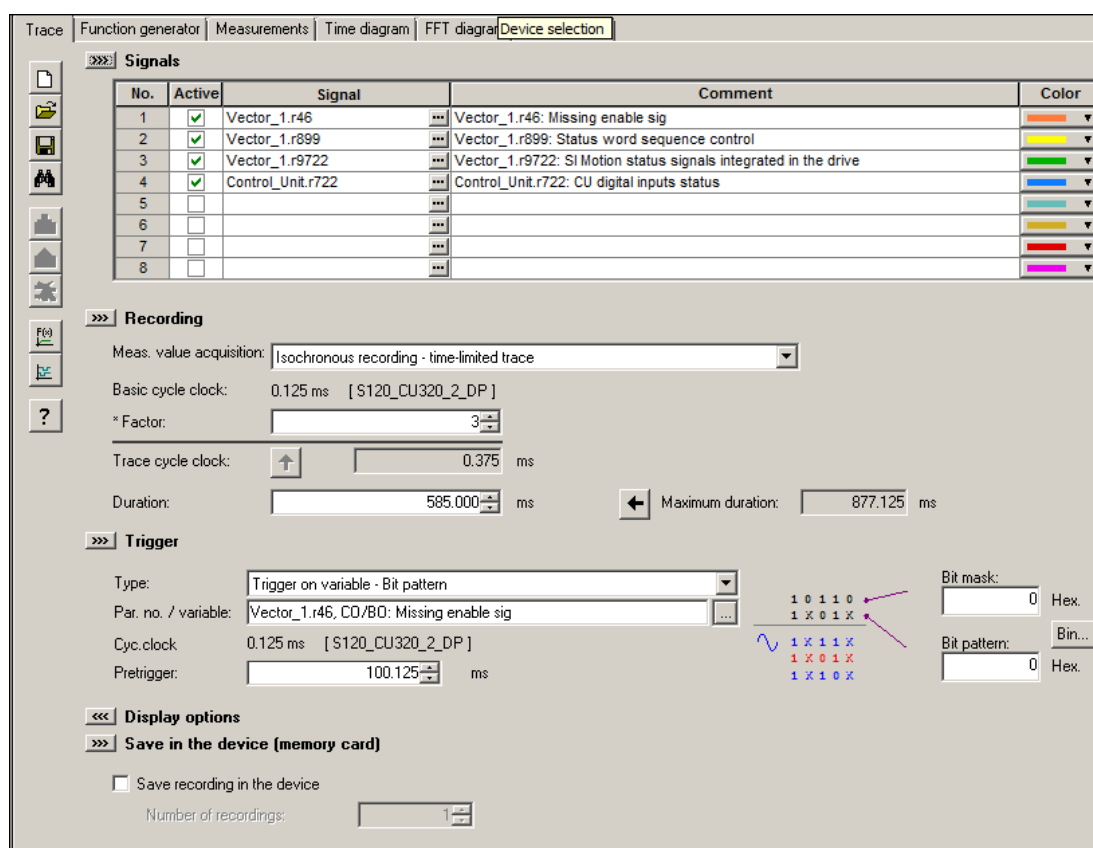
Изображение 4-8 Запуск трассировки в STARTER
