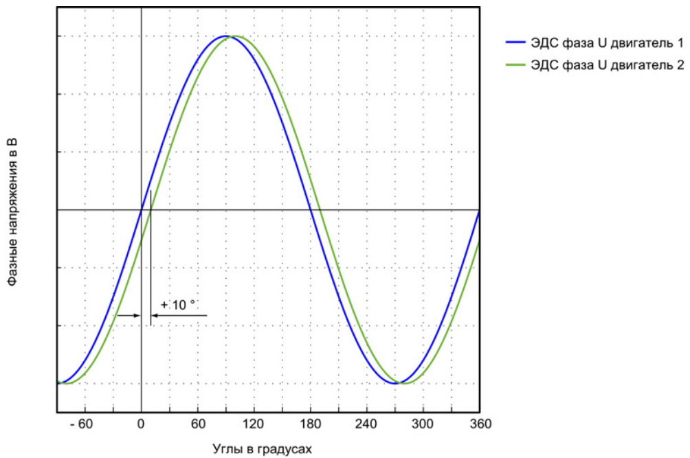
Изображение 3-59 ЭДС фаза U двигателя 1 может опережать ЭДС фаза U двигателя 2 не более чем на 10^\circ
