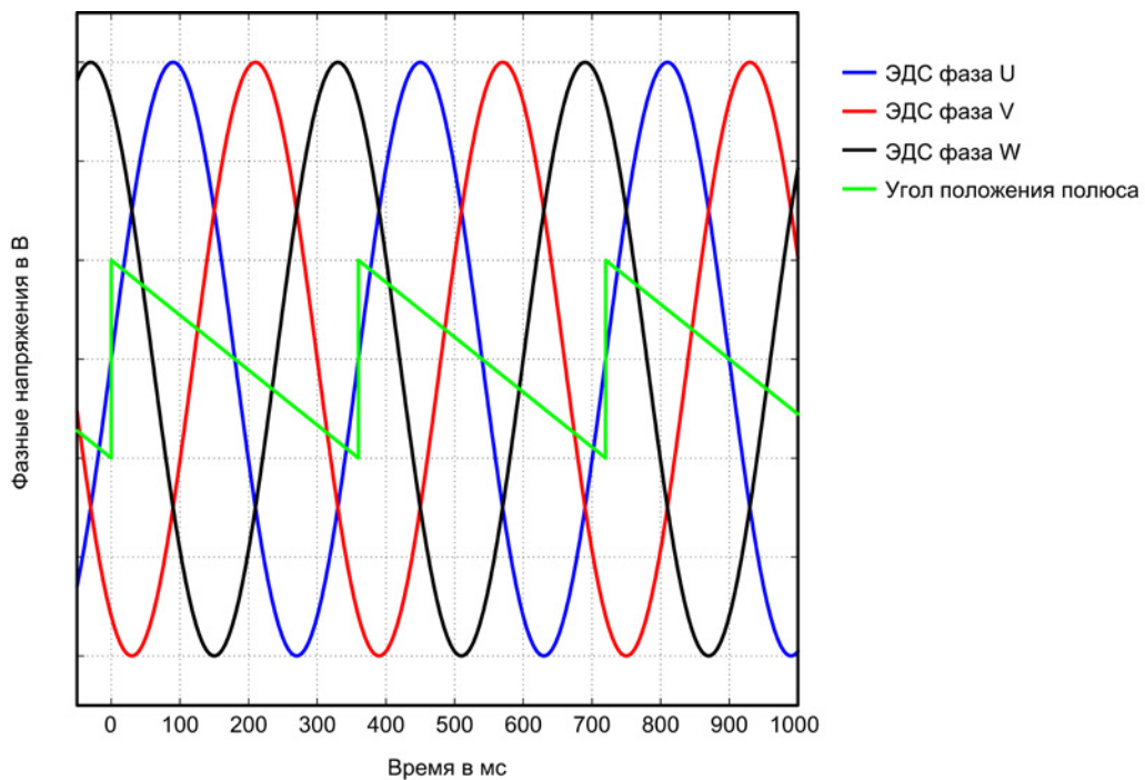
Изображение 3-93 ЭДС при неправильном инвертировании фактического значения частоты вращения
